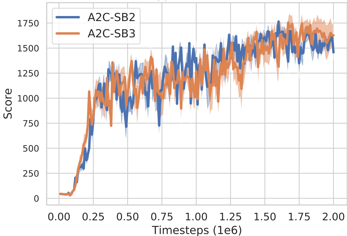
HopperBulletEnv-v0
