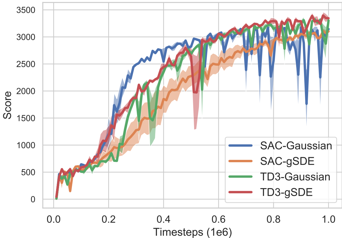
AntBulletEnv-v0
