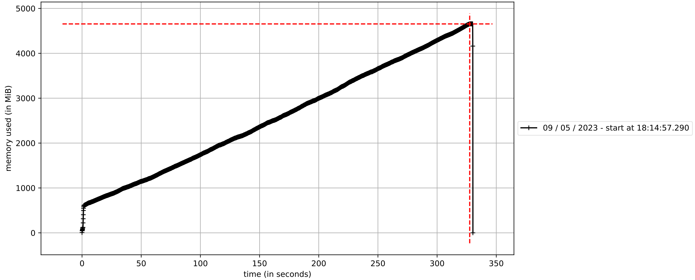
pymatgen v2023.5.8
